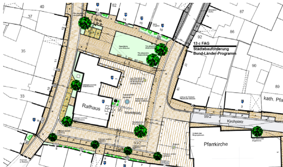
Marktplatzneugestaltung - © Arch. Schröder, Schweinfurt
