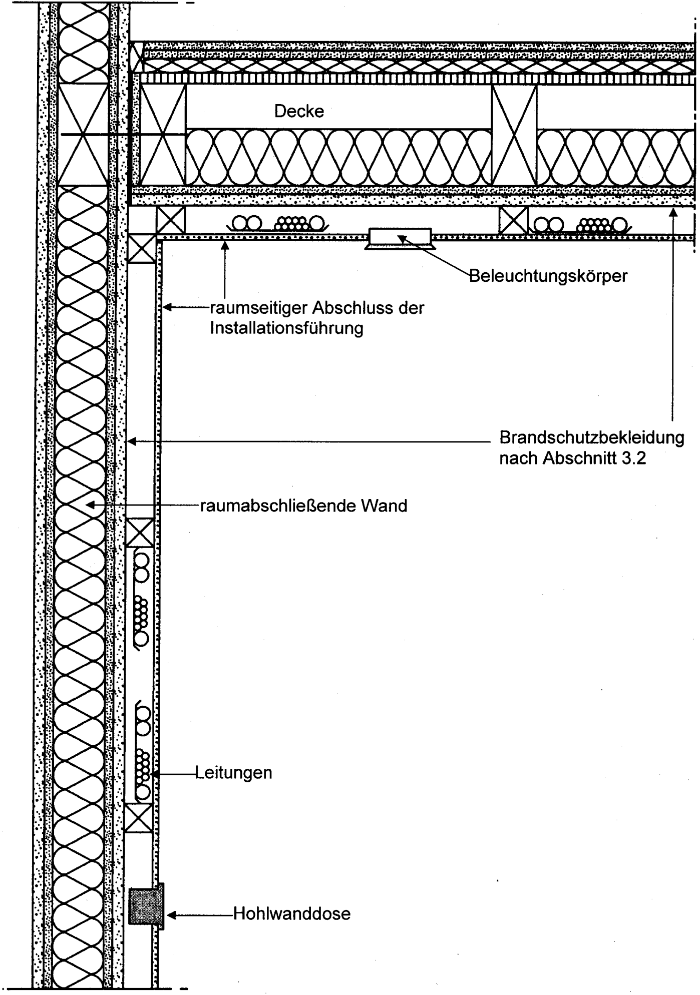
Bild 8 Installationsführung
