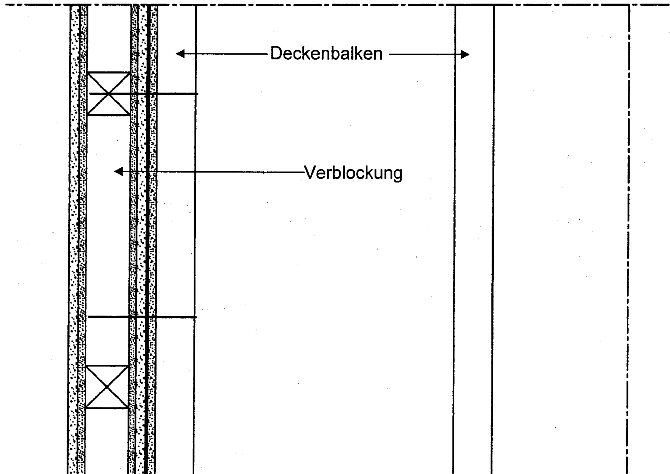
Bild 2 Anschluss Decke nach Abschn. 3.3.3 an durchlaufende raumabschließende Wand nach Abschn. 3.3.2 (Treppenraumwand, Außenwand, auch nichttragend – Spannrichtung der Deckenbalken parallel zur Wand)
